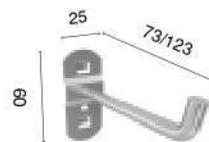
НК/НК-3 Крючок L = 7 / 12 см
