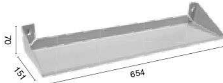
TH Держатель инструмента
