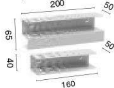
Держатели для шестигранников и сверл
